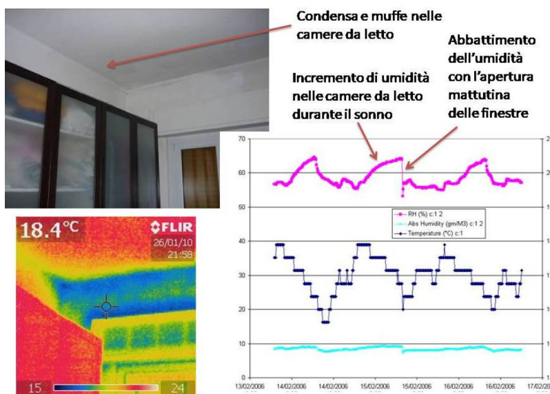
Fig. 1: Grafico dell'andamento dell'umidità in una camera da letto e effetti di degrado
