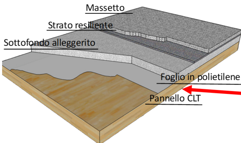
Fig. 1: Massetto galleggiante
