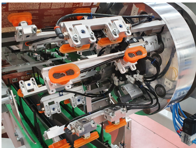
Fig. 1: Gruppo camma prototipo
