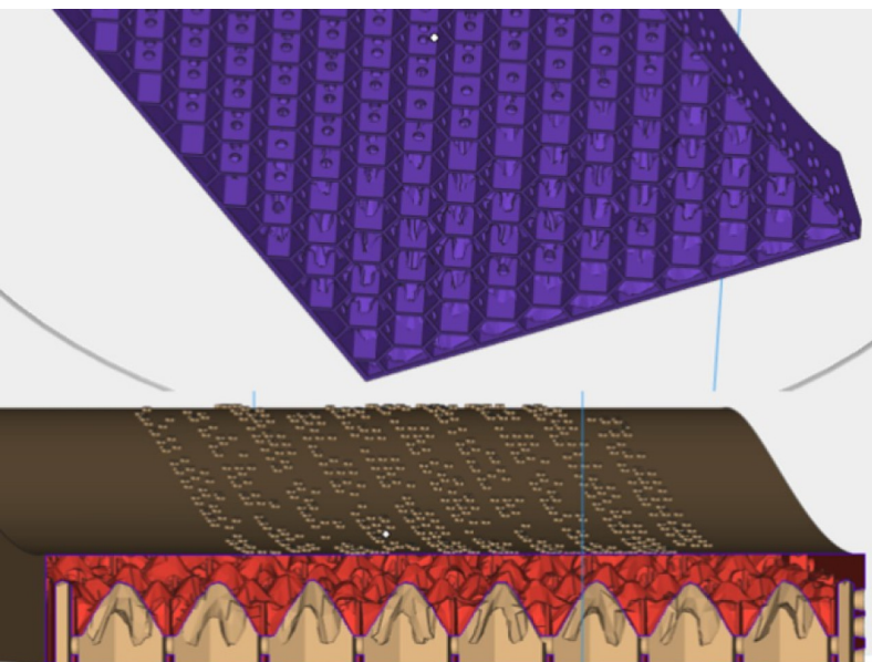
Fig. 3: Alloggerimento strutturale autoportante interno. Braille applicato alla superficie esterna
