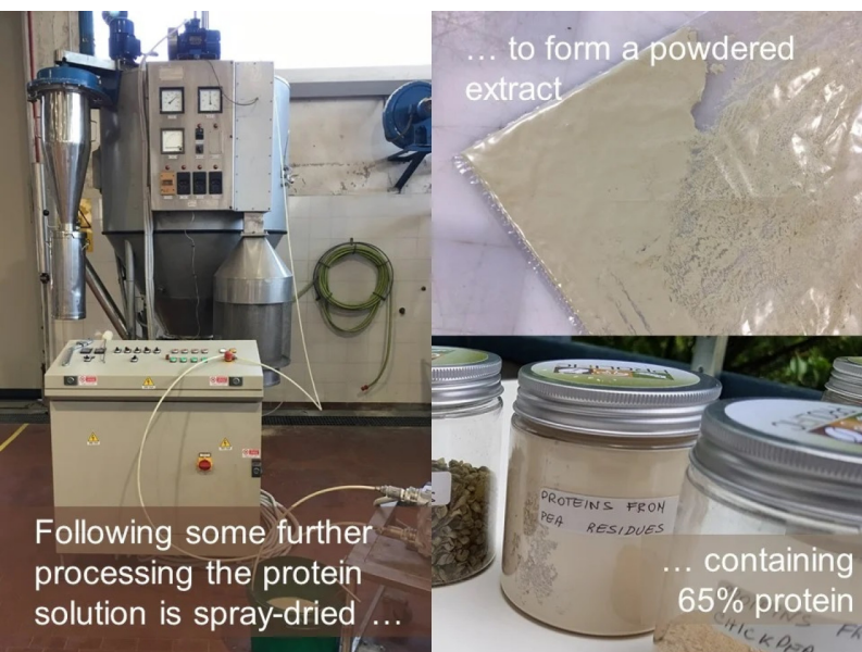
Fig. 3: Concentrati proteici da sottoprodotti della filiera dei legumi (piselli, ceci e lenticchie)
