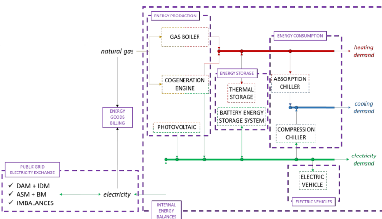
Fig. 2: Caso studio PoliMi – Il rapporto simbiotico reti-distretto
