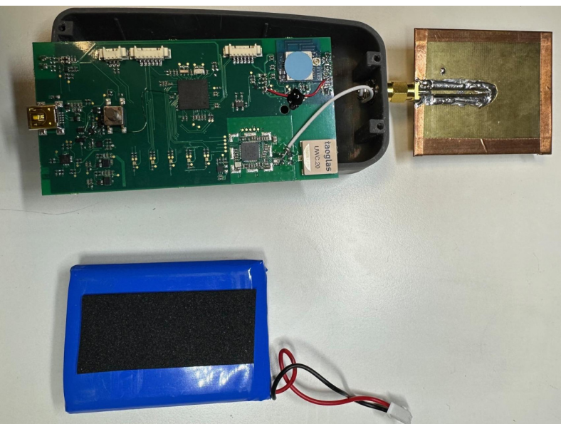
Fig. 3: Prototipo di sensore a batteria per misura posizione e prestazioni degli atleti
