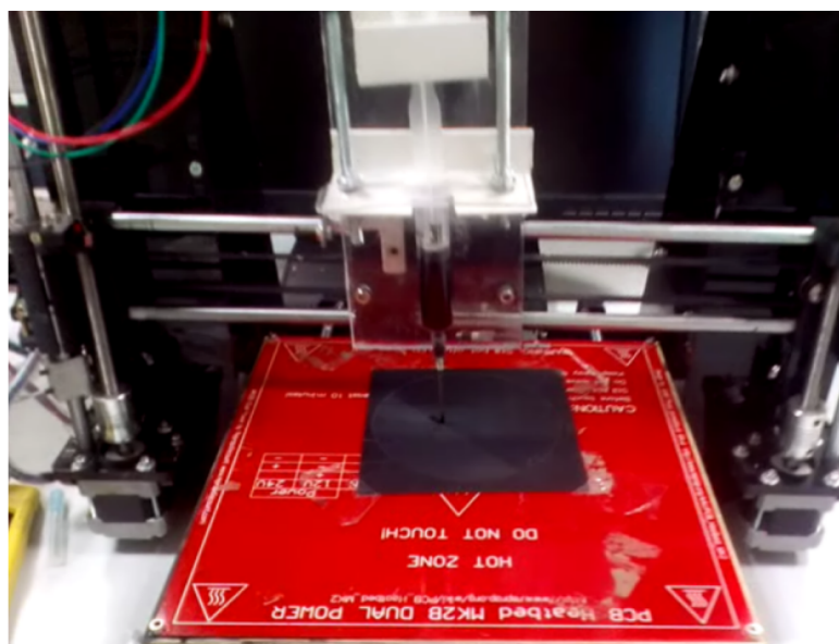
Fig. 1: Stampante 3D modificata per la deposizione di inchiostri catalitici per PEMFC. Vers. 2.0
