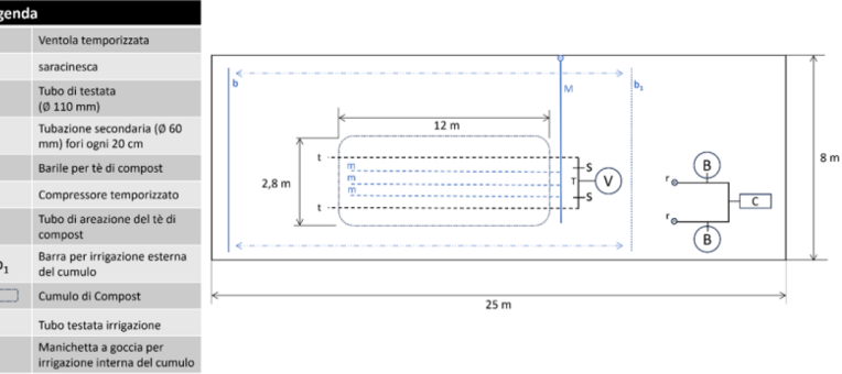
Fig. 2: Schema della serra dove è stata posizionato l'impianto pilota.
