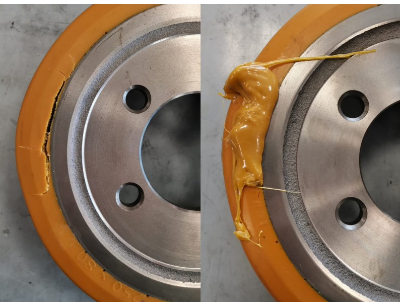
Fig. 2: Esempi di rottura: a) Fessurazione agli estremi della fascia di attacco al mozzo; b) Fusione del poliuretano.
