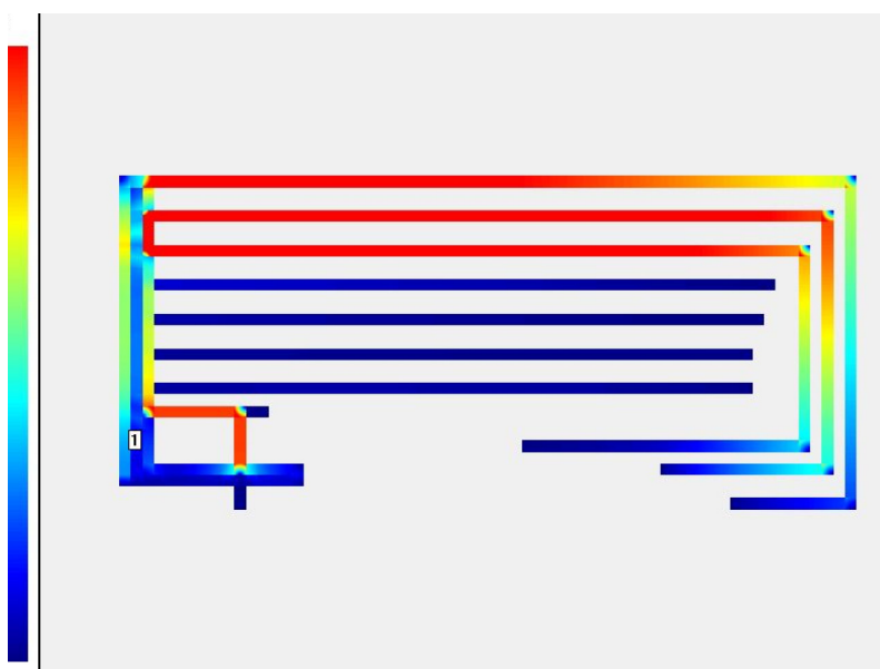
Fig. 1: Antenna interdigitata: 600 MHz 2,5 GHz (simulazione elettromagnetica dell'andamento della corrente)
