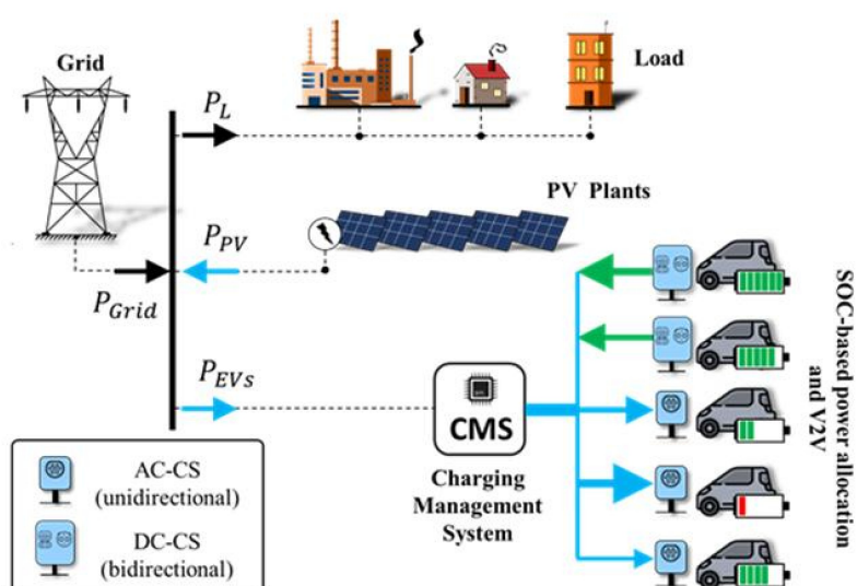
Fig. 1: Schema di un distretto energetico con sistema di gestione (CMS) delle stazioni di ricarica (CS)
