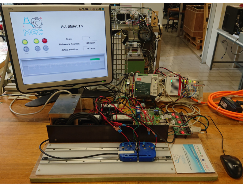
Fig. 3: Act-SMART, l'azionamento SMA innovativo di ACMEC collegato via EtherCAT, come asse elettrico custom, ad un PLC Beckhoff.
