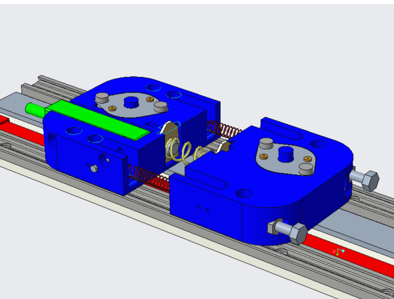
Fig. 2: Progetto di movimentazione rettilinea a "bruco". L'attuazione si ottiene scaldando e raffreddando la "molla" SMA al centro in combinazione con l'attivazione ragionata dei freni sulle rispettive teste.
