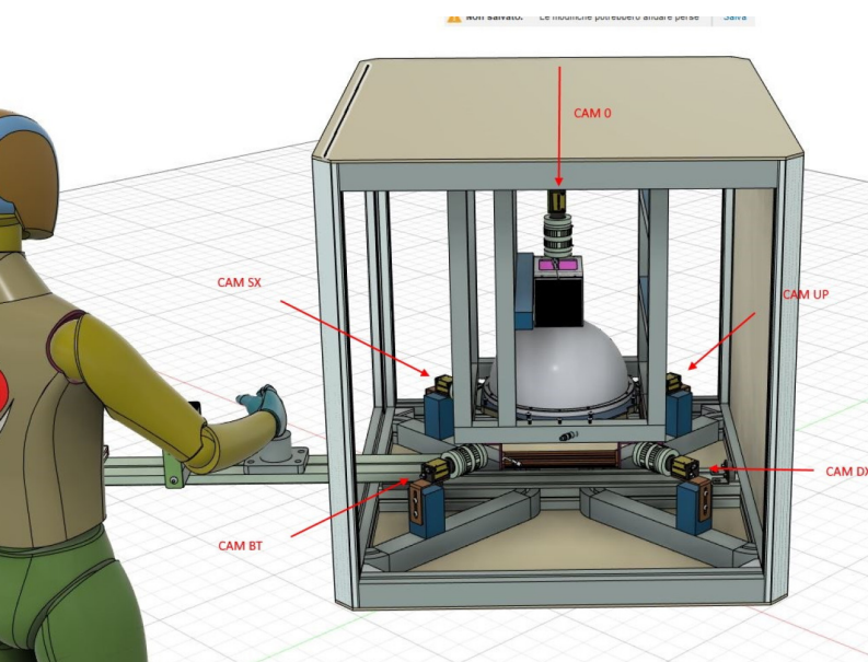
Fig. 2: Struttura a CAD della camera di visione
