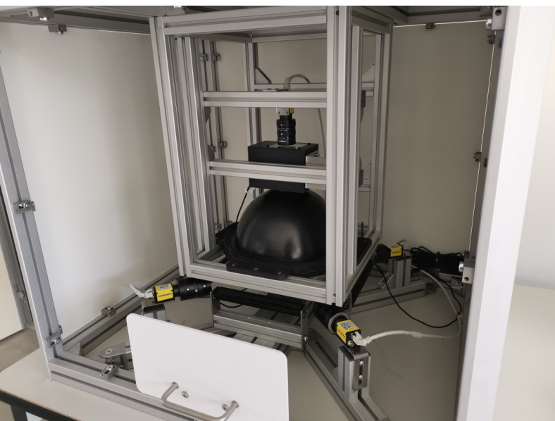
Fig. 3: Sistema di Visione per Controllo Qualità Componenti - APERTO. Si può notare la struttura del sistema con le 4 telecamere alla base e quella all'apice soprastata da un illuminatore a cupola.
