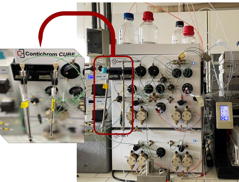
Fig. 2: Strumentazione per cromatografia preparativa in continuo dotata di due colonne cromatografiche
