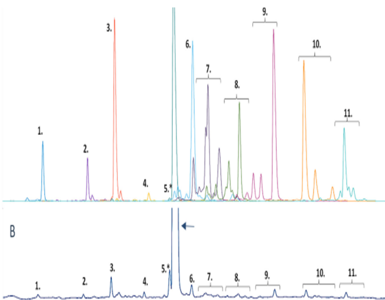
Fig. 3: Confronto tra il cromatogramma analitico della miscela complessa (feed) e delle frazioni arricchite nei componenti minoritari grazie a processi cromatografici multicolonna
