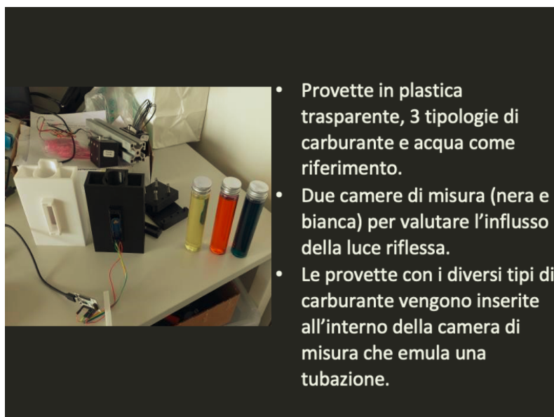
Fig. 1: Camera di misura con sensore.
