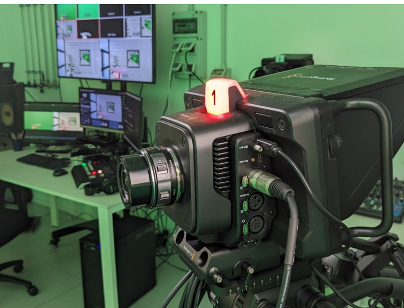
Fig. 2: Telecamera Blackmagic Design 4K e postazione di regia
