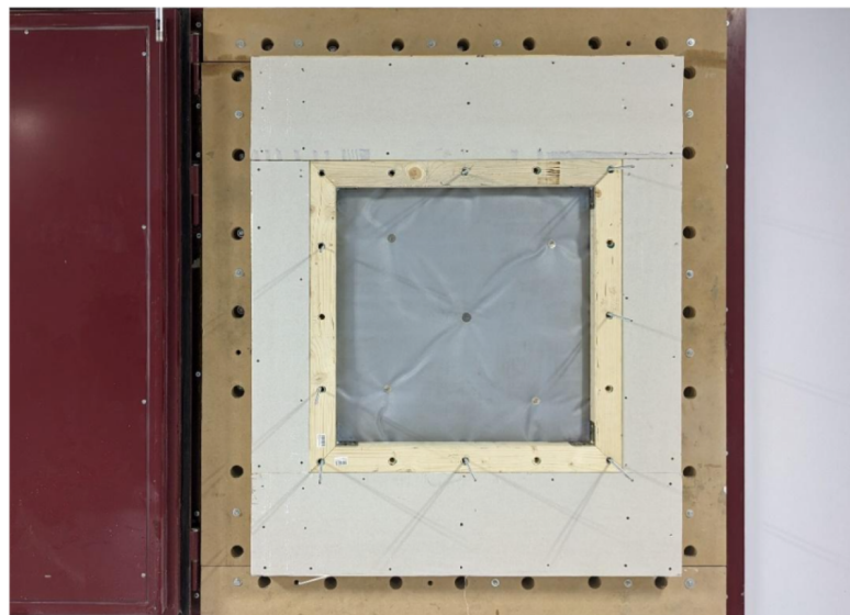
Fig. 3: Setup di misura delle prestazioni di isolamento acustico del sistema di mitigazione acustica nella Camera Riverberante del Dipartimento di Ingegneria dell'Università di Ferrara
