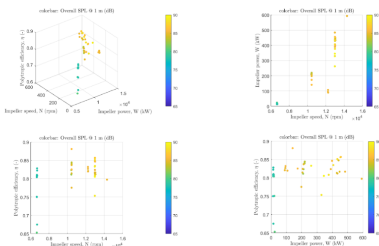
Fig. 1: Analisi statistica dei livelli di pressione sonora misurati sperimentalmente in relazione ai parametri di macchina
