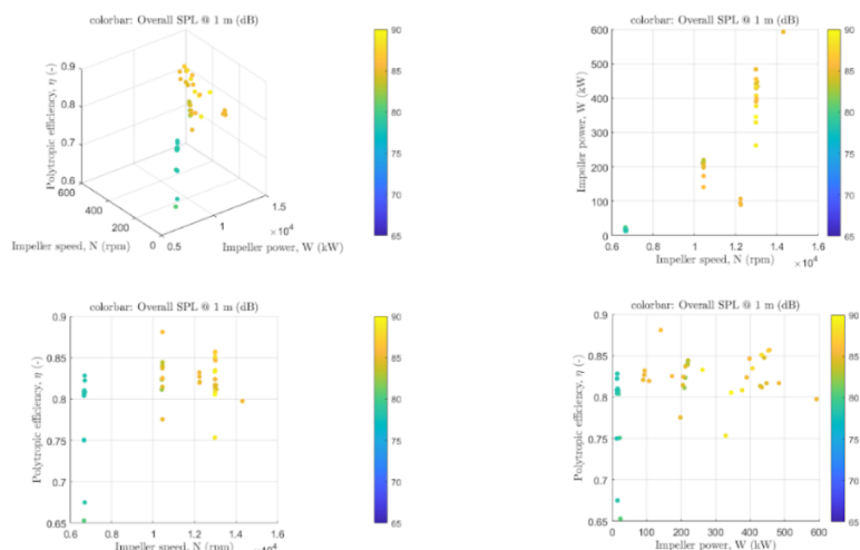
Fig. 2: Analisi statistica dei livelli di pressione sonora misurati sperimentalmente in relazione ai parametri di macchina
