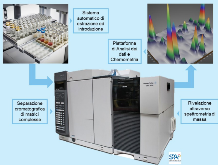
Fig. 2: Piattaforma di estrazione, analisi cromatografica, identificazione dei composti aromatici e statistica
