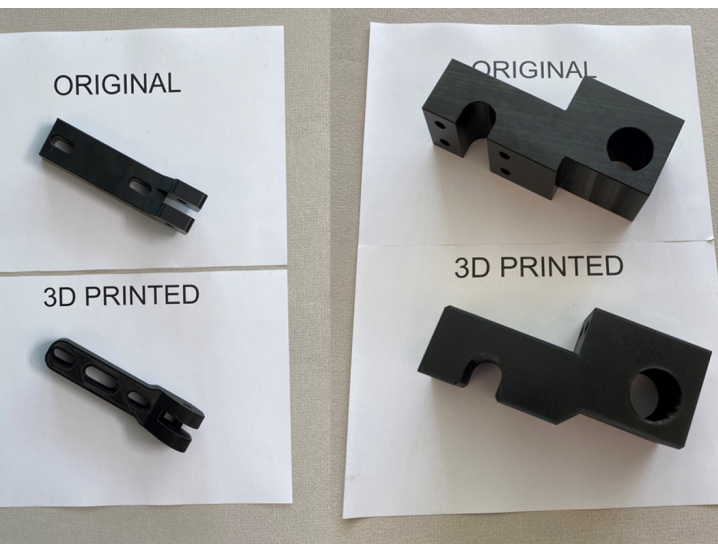
Fig. 3: Confronto tra componenti realizzati con tecniche tradizionali e con tecnologie AM
