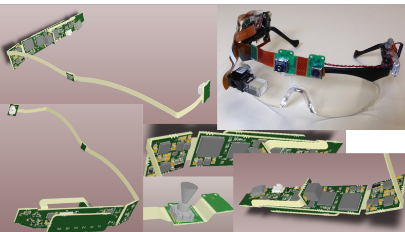
Fig. 3: Esempi di simulazioni meccaniche ed elettriche del PCB
