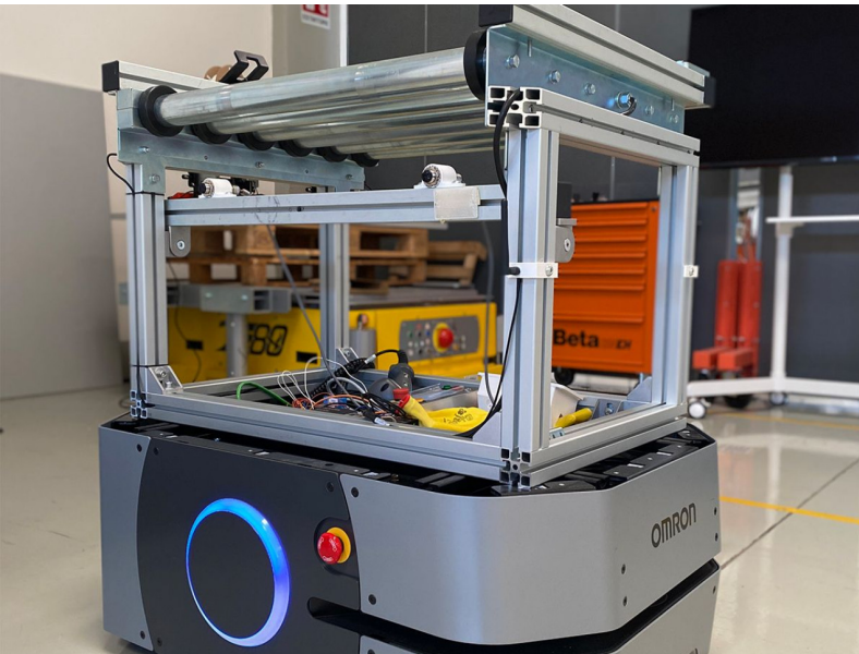
Fig. 2: Test AMR con rulliera custom
