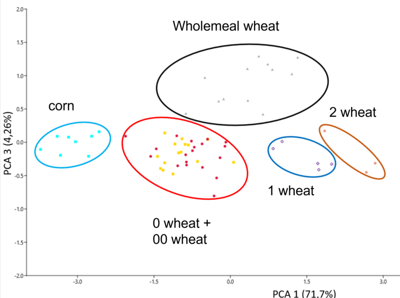
Fig. 3: Analisi statistica utilizzando i dati ottenuti dall'ICP-MS-QQQ: le farine di grano si differenziano in base alla presenza degli elementi diversi a seconda del grado di macinazione.
