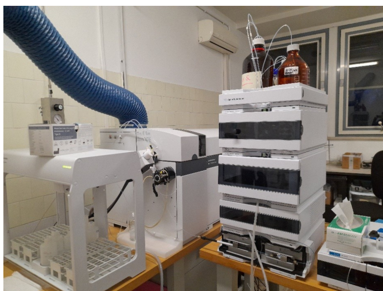
Fig. 1: Sistema HPLC bio-inert accoppiato a ICP-MS
